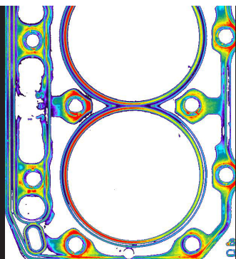
GASKET
